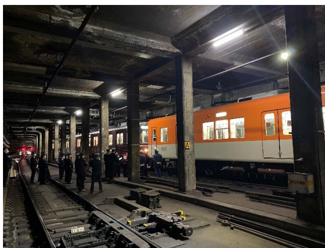
三社合同推進運転訓練 2024年12月1日（新開地駅・高速神戸駅間にて）
